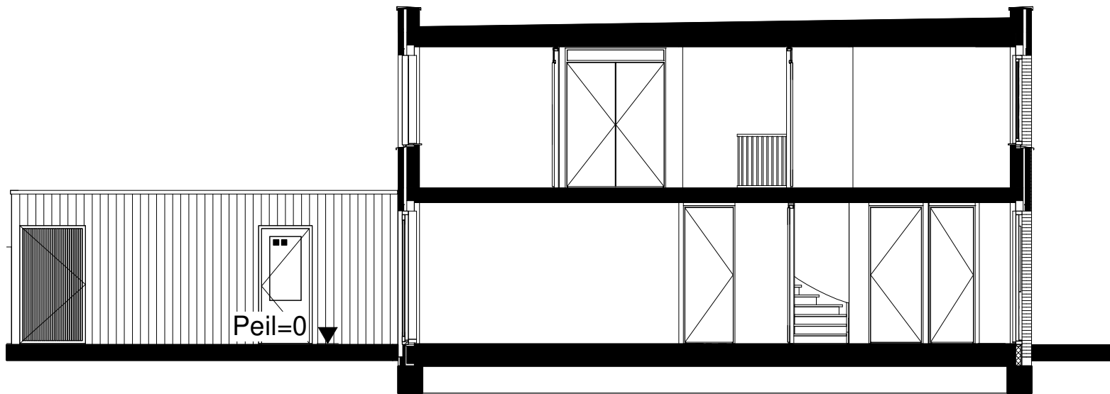
doorsnede
