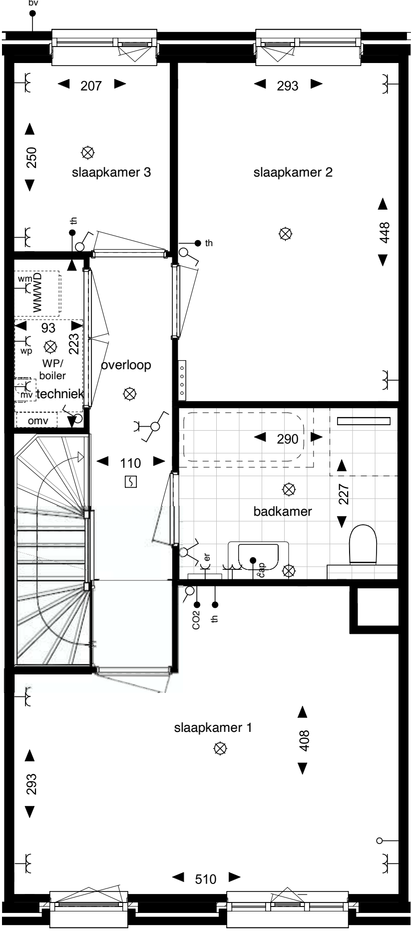
eerste verdieping BNR 54, 56
