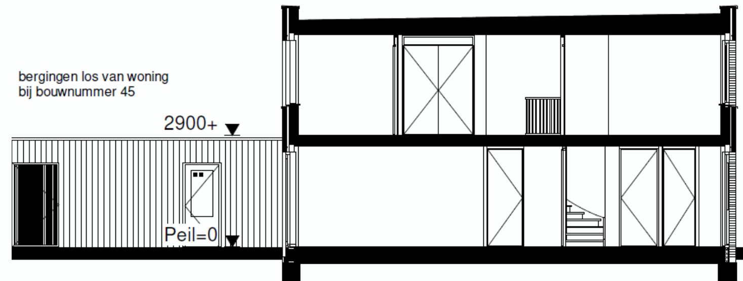
doorsnede
