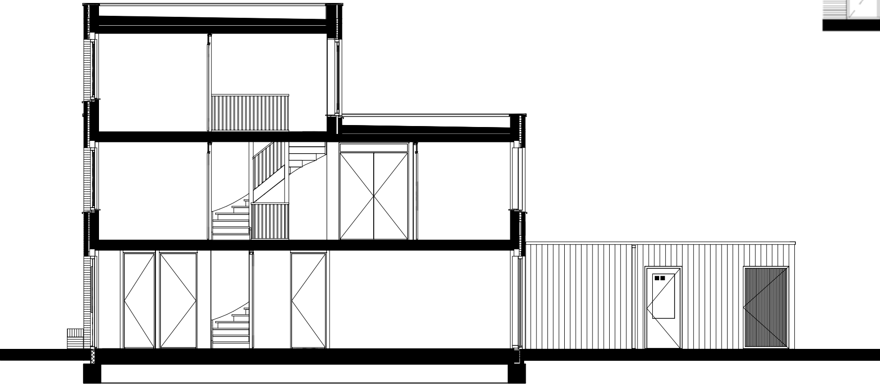
doorsnede
