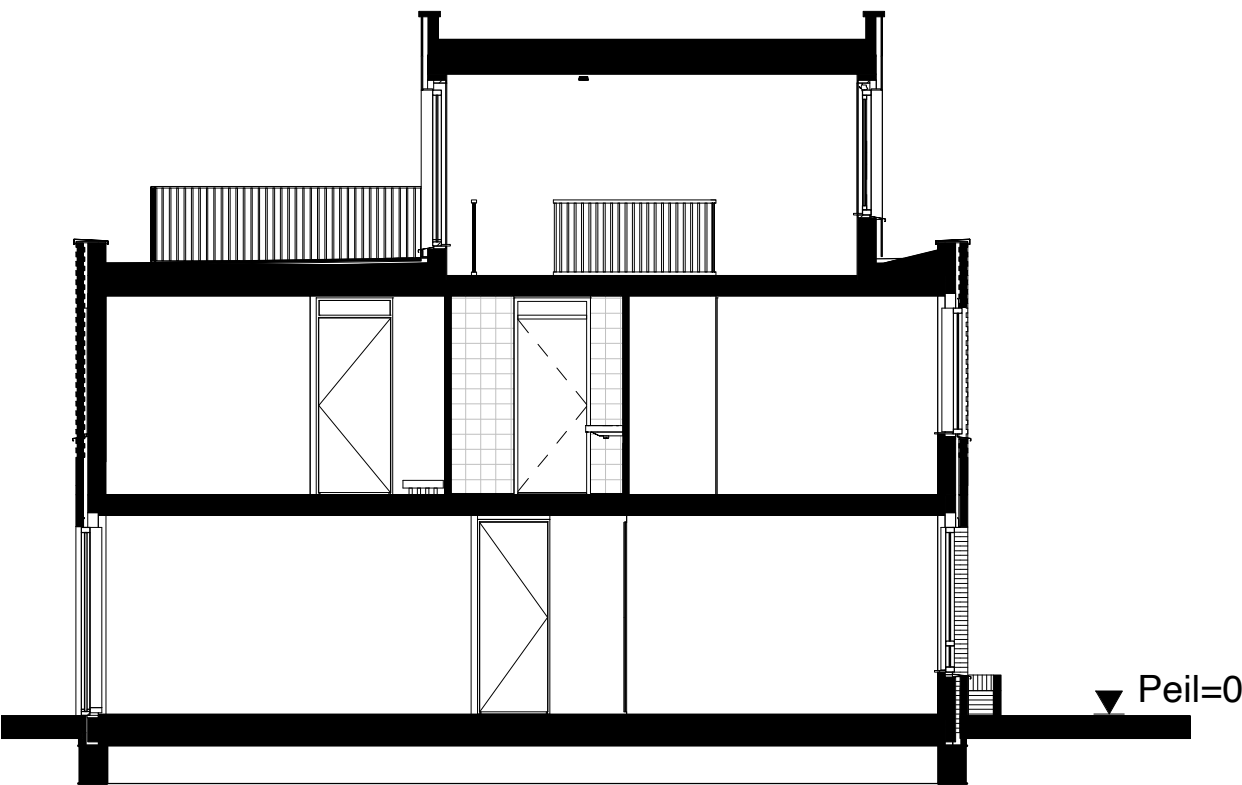
doorsnede
