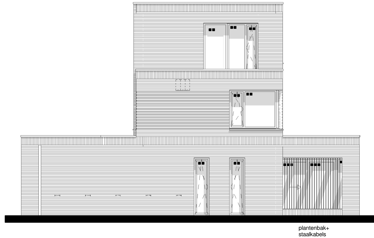
rechter zijgevel
