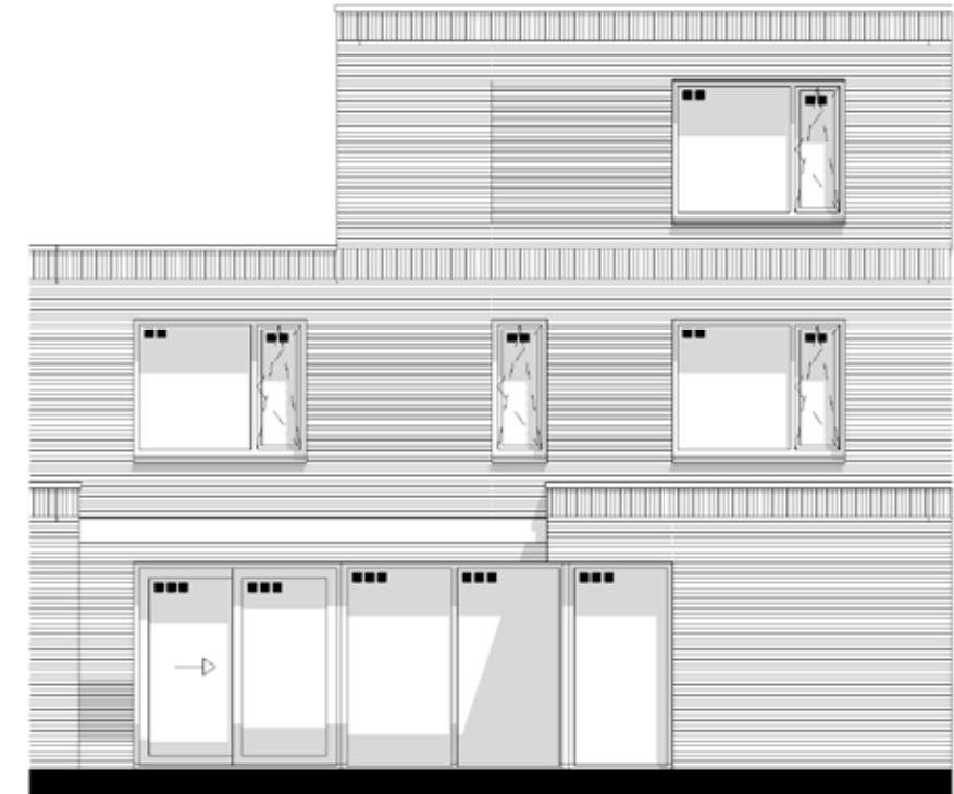
achtergevel
