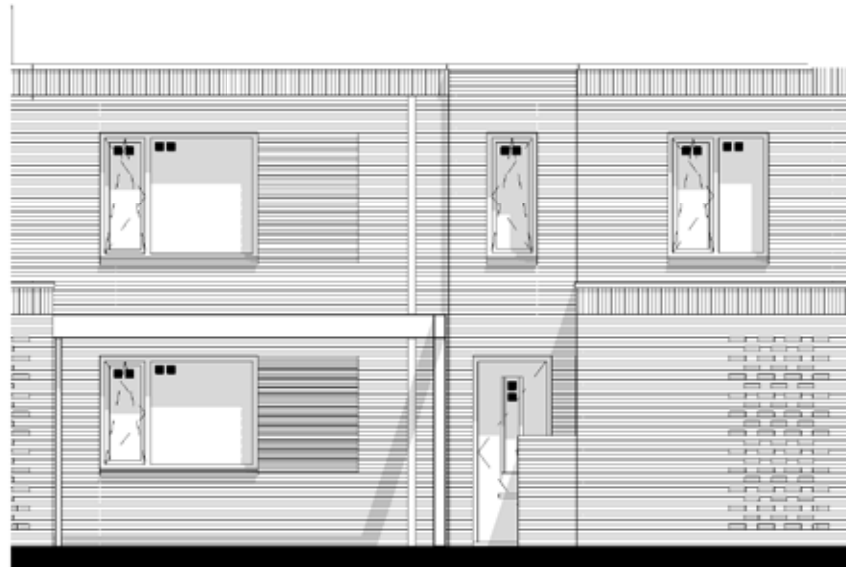
voorgevel
