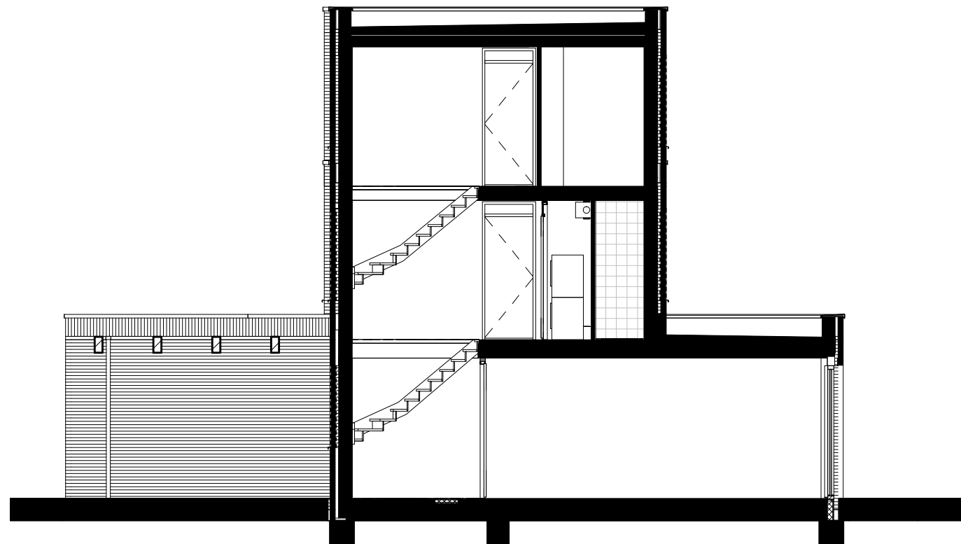
doorsnede
