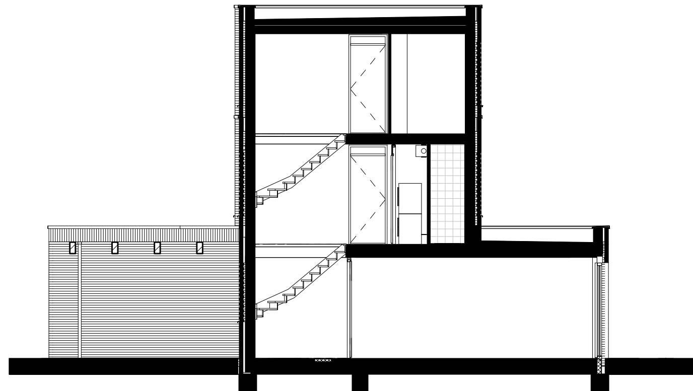
doorsnede
